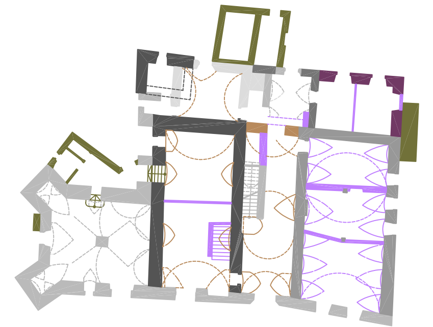
Bauphase 9 Bauphasen Erdgeschoß
